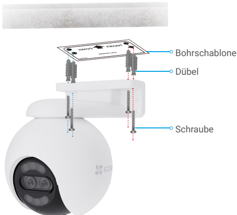
Abb. 1 Deckenmontage
